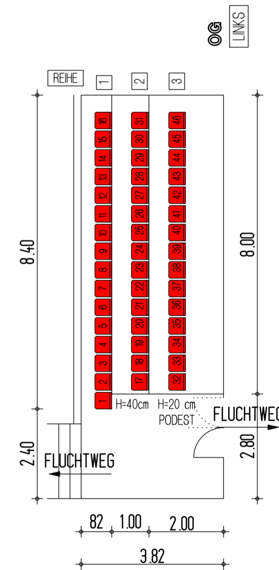
SITZPLAN OBERGESCHOSS
