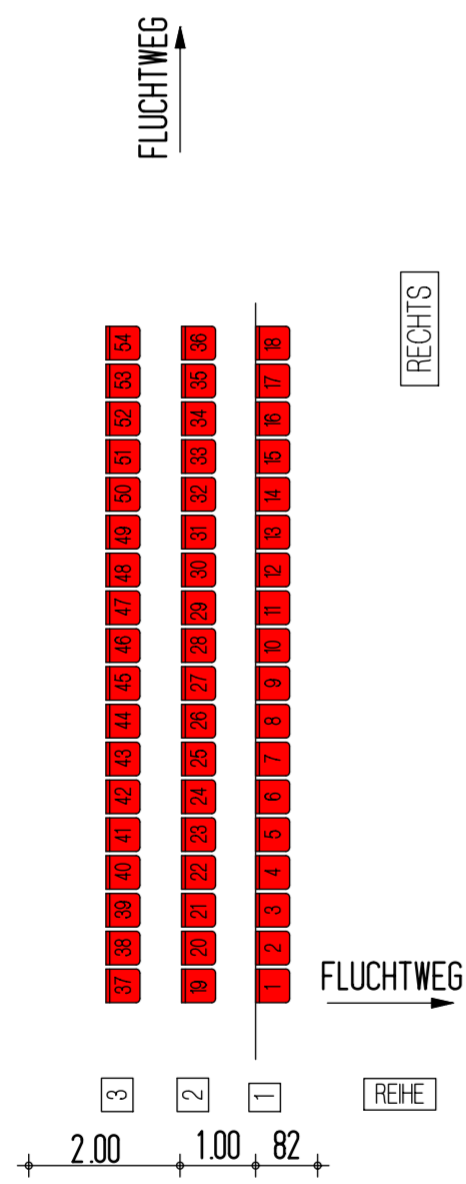
SITZPLAN OBERGESCHOSS
